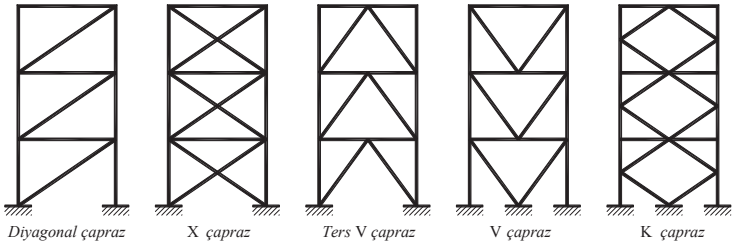
Şekil 4.4. Merkezi Çelik Çaprazlı Perdeler
