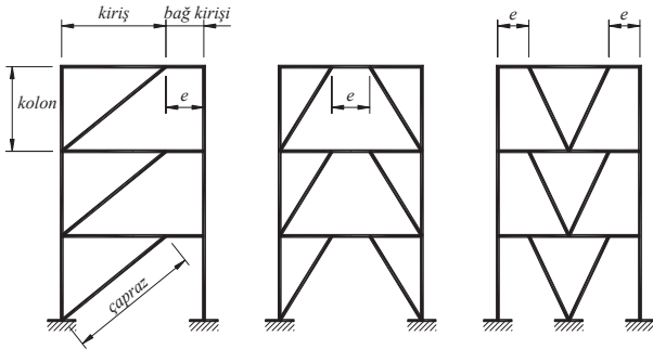
Şekil 4.5. Dışmerkez Çelik Çaprazlı Perdeler
